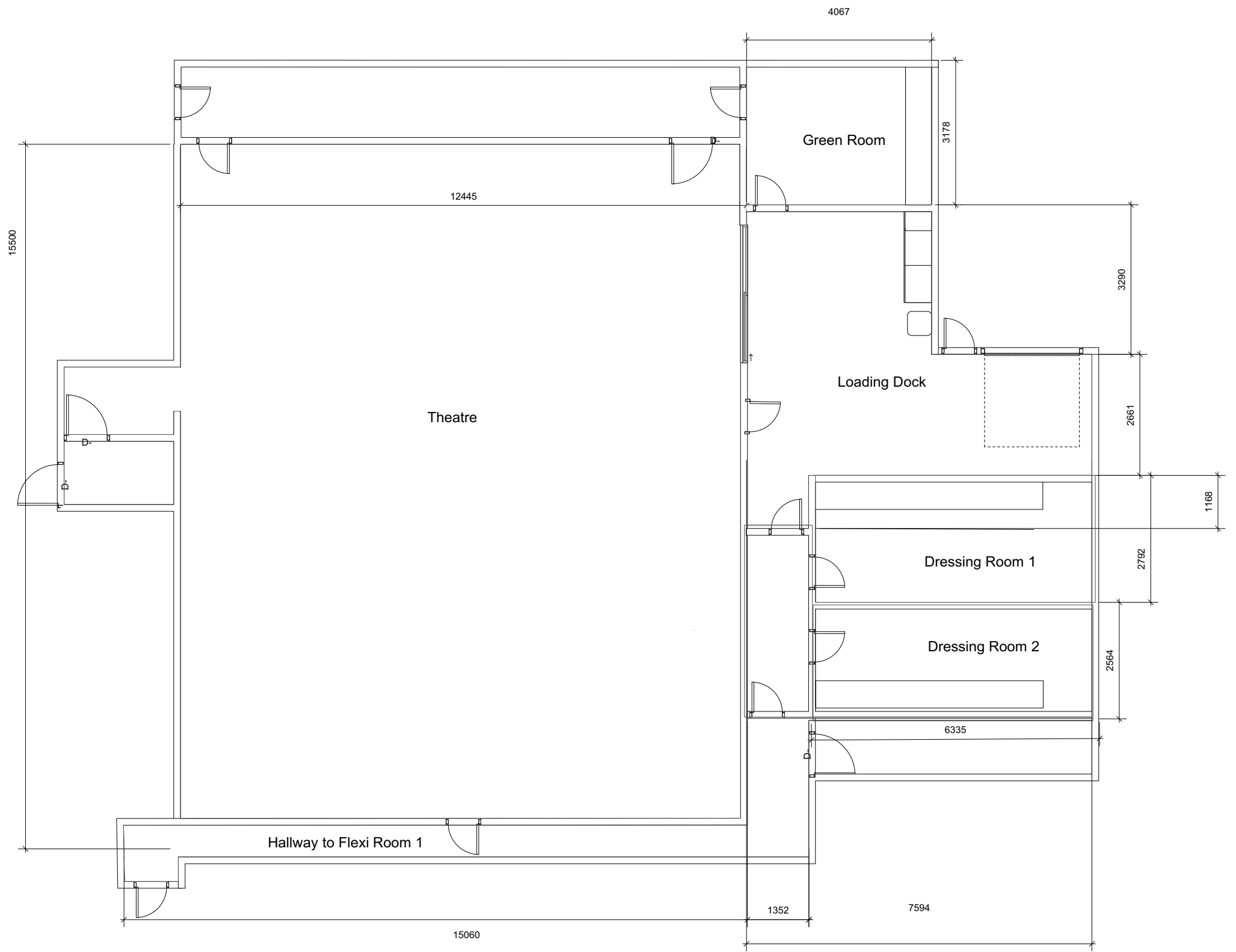
1 Theatre Scale: 1:50
